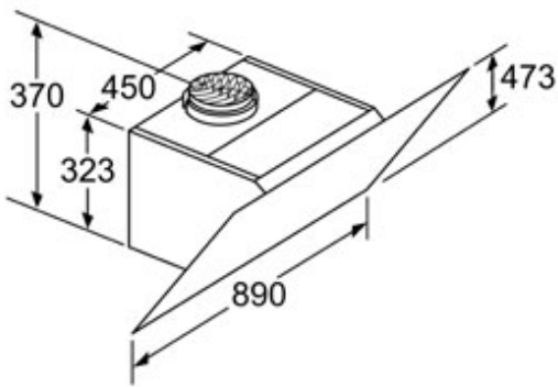
Aparato en recirculación de aire sin canal Será necesario un juego de recirculación de aire Dimensiones en mm
