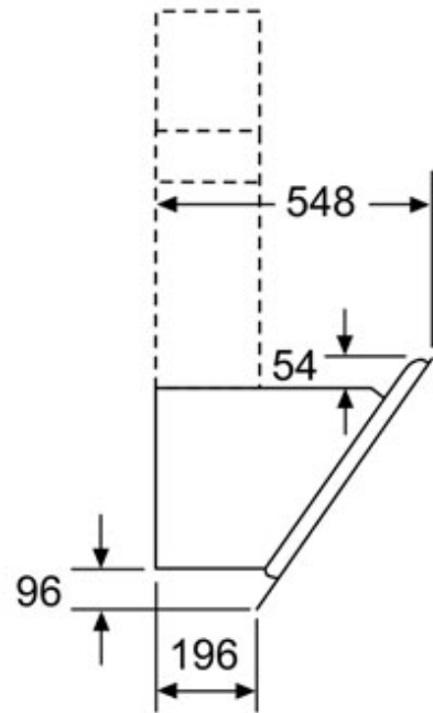
Dimensiones en mm
